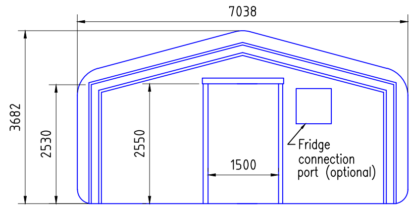
DOOR ELEVATION
